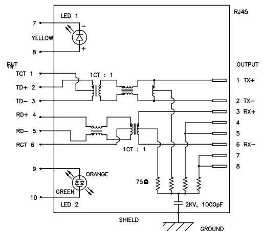
Schematic 9L
