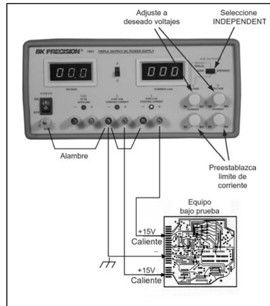
Fig. 12. Conexión típica usando dos voltajes positivos diferentes y un negativo común
