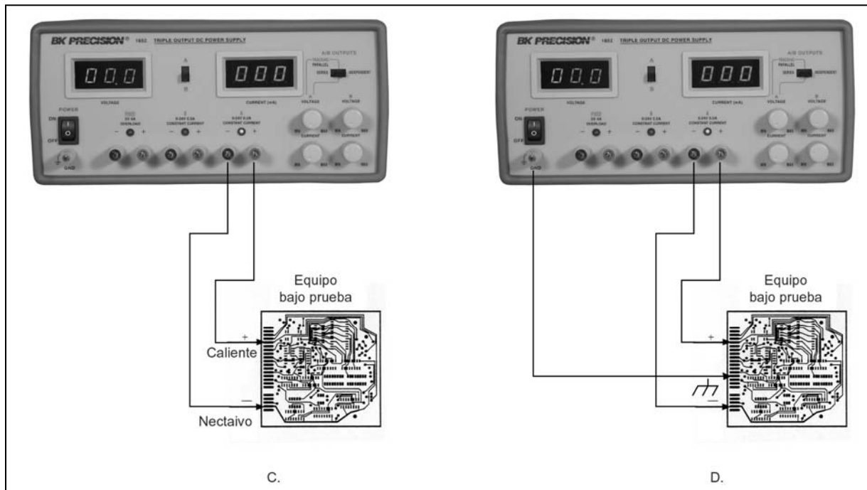
Fig. 9. Posibilidades de conexión a tierra en operación de rastreo en paralelo (2 de 2)
