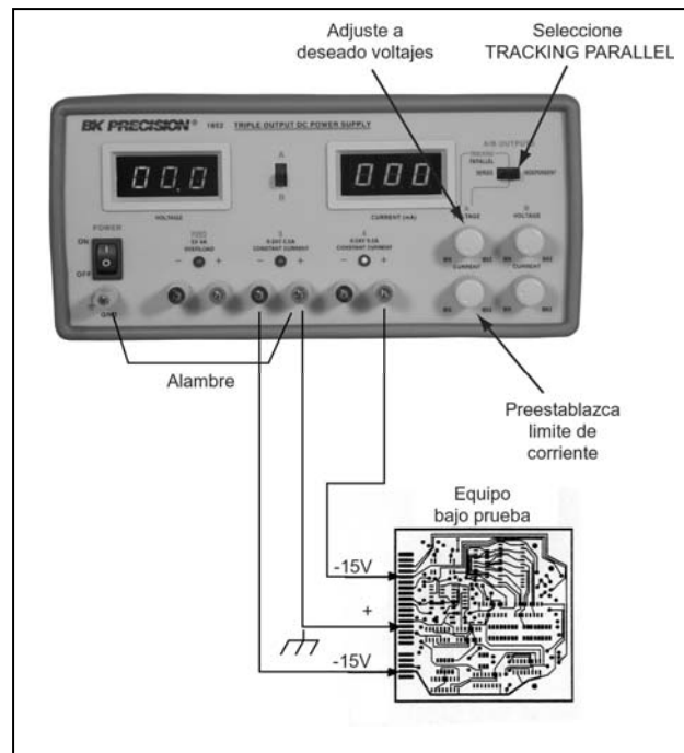
Fig. 13. Conexión típica usando dos voltajes negativos diferentes y un positivo común
