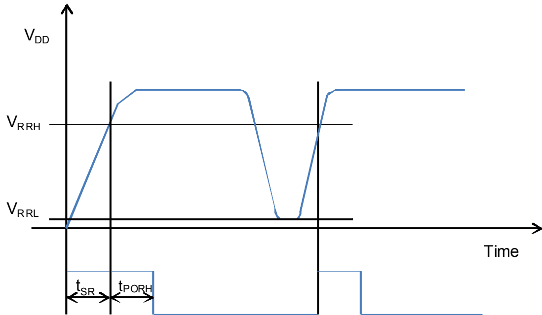
Figure 21.5. POR Timing Diagram
