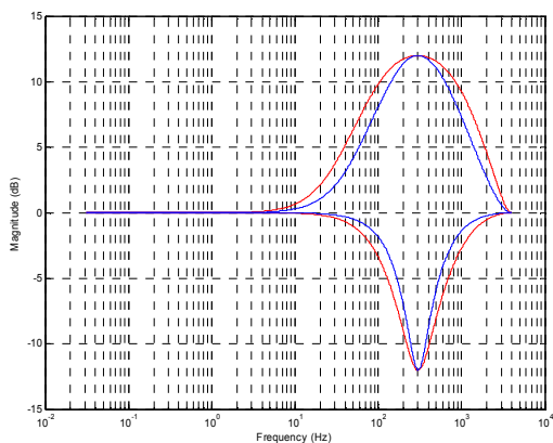
Figure 61 EQ Band 4 – EQ3BW=0, EQ3BW=1
