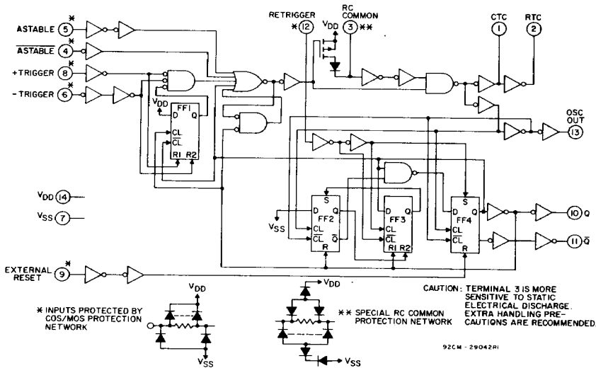
Fig. 2—CD4047B logic diagram.
