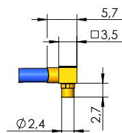
MMPX™-m (angular 90°)
