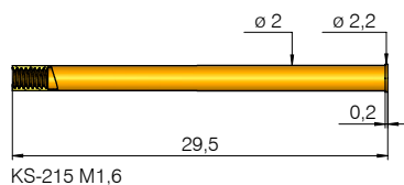
KS-215 M1,6
