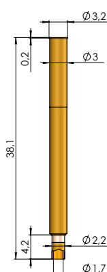
KS-465 M2,5-F
