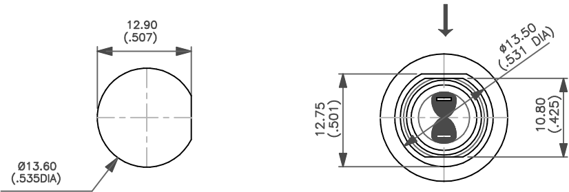
DECOUPE DU PANNEAU PANEL CUT-OUT
