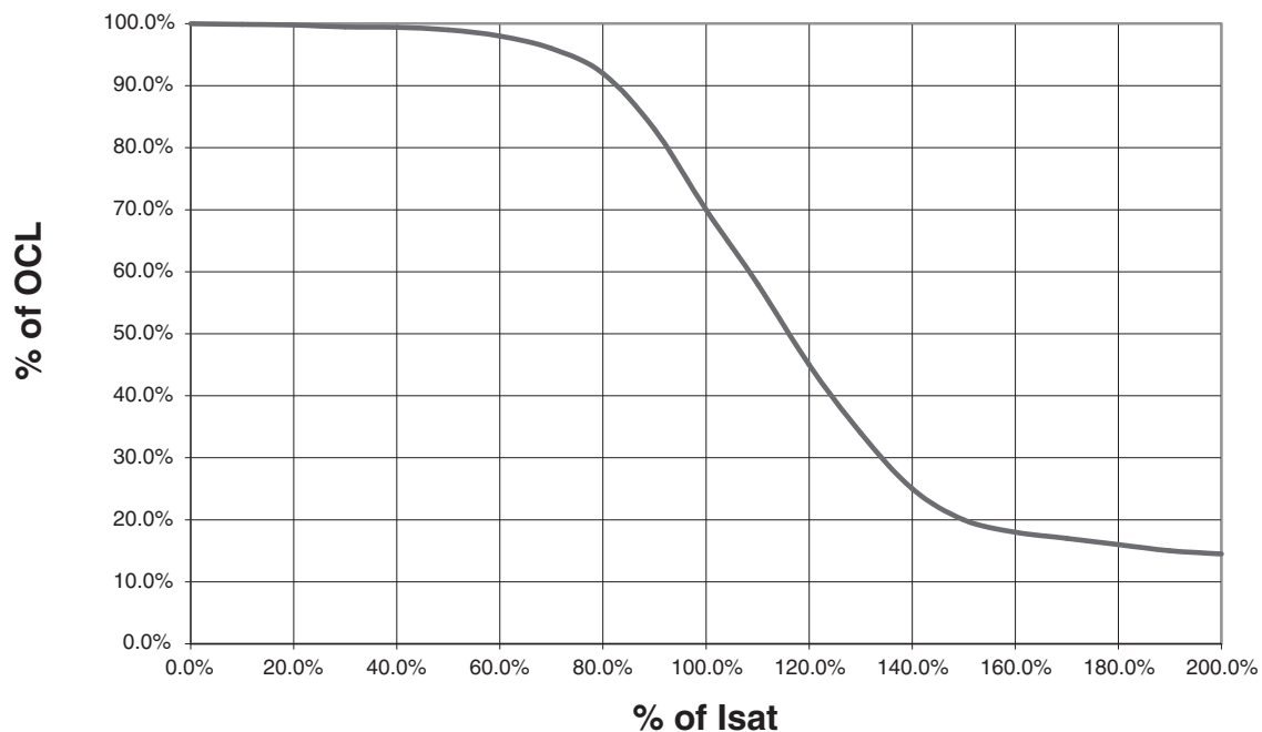
OCL vs. Isat
