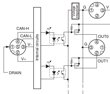
DRT2-WD16CL-1 (PNP)
