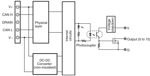
DRT2-OD16ML(X)
