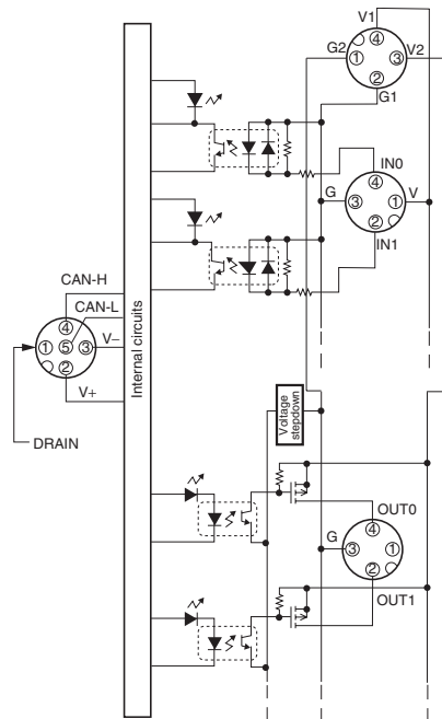
DRT2-MD16CL-1 (PNP)
