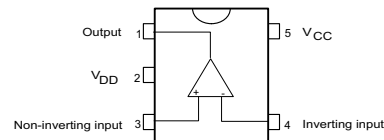
TS971ID-TS971IDT (SO-8)
