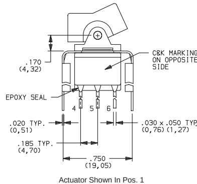
E201J1_BE2 DPDT
