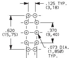
E201J1_BE2 DPDT
