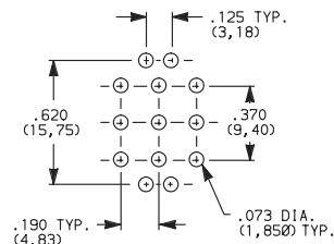
E301J1_BE2 3PDT
