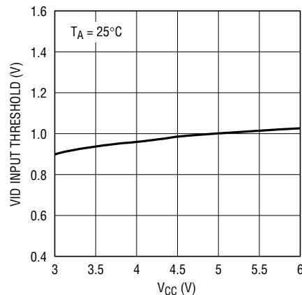
VID Input Threshold vs V_{CC}
