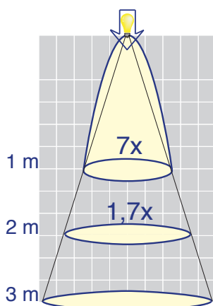
PL119940 (30°) - 2 METER
