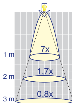
PL119940 (30°) - 3 METER
