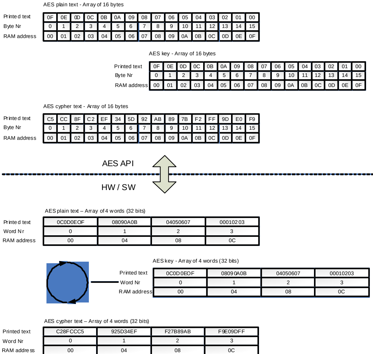
Fig 27. AES endianness
