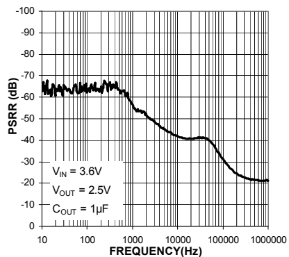
LDO2 PSRR ( I_{\text{OUT}} = 150\text{mA} )
