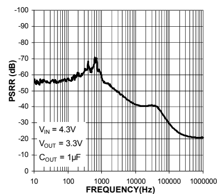
LDO1 PSRR ( I_{\text{OUT}} = 150\text{mA} )
