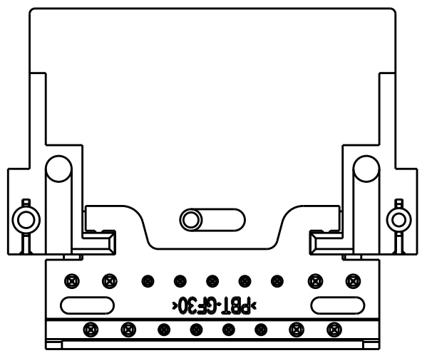
638134-4, -6 KEY B
