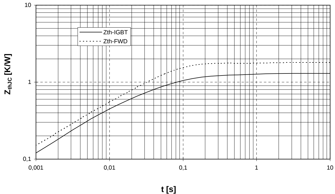
Transienter Wärmewiderstand Wechslr.
