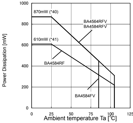
(d)BA4564R/BA4584/BA4584R family
