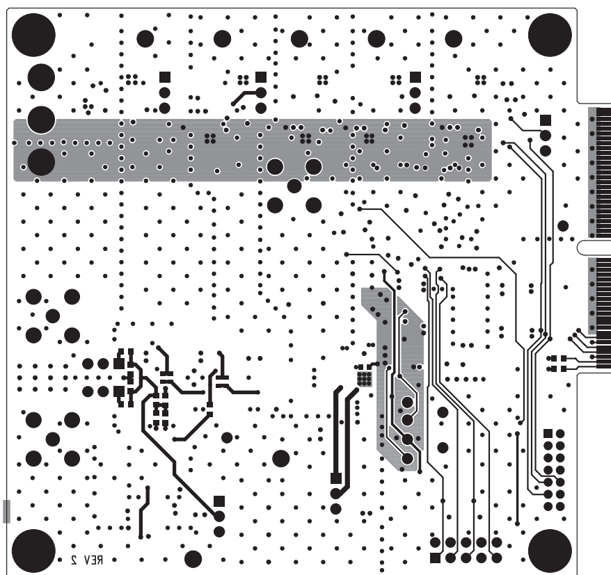
Layer 4 Bottom Layer
