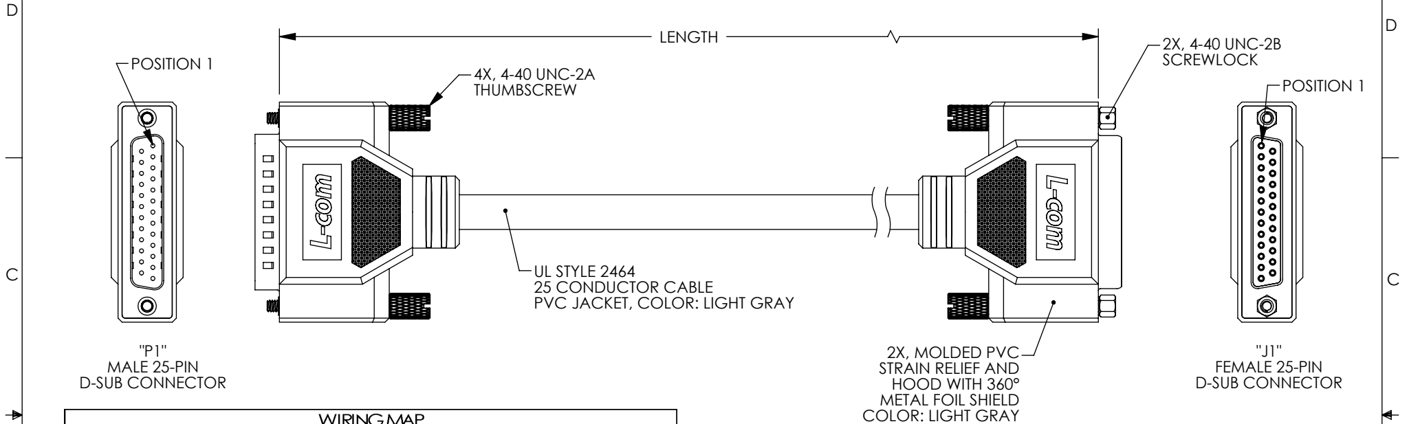
WIRING MAP
