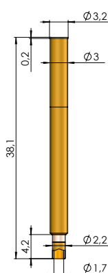
KS-465 M2,5-F
