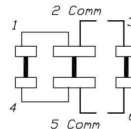
CIRCUIT: SPDT
