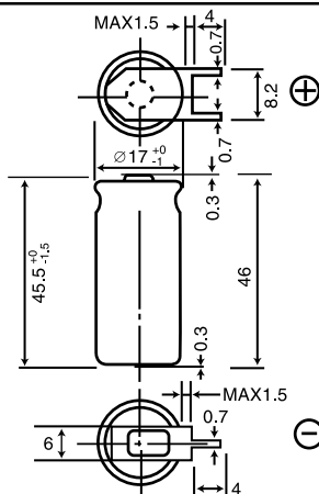
BR-AE2P BR-AGE2P*
