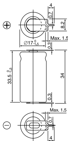
BR-2/3AE5SP BR-2/3AGE5SP*
