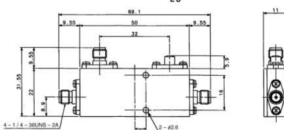
HDH-02220AID(40)
