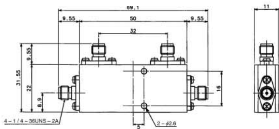
HDH-02210AI(40) HDH-02249AI(40)
