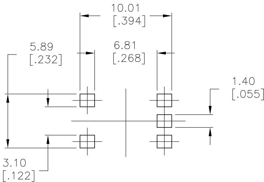
P.C.B. FOOTPRINT
