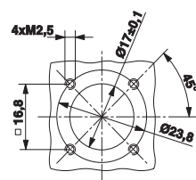
Einbaumaße: ST-17.1N8AAD00S
