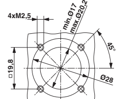
Einbaumaße: ST-17.1N8AAC00S
