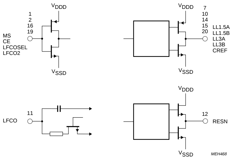
Fig.5 Internal circuit.
