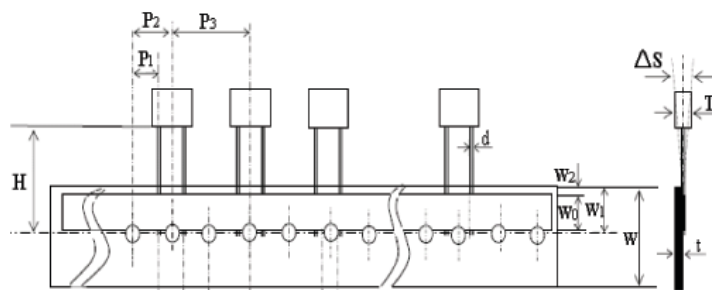
Fig.2 P=10.0、15.0mm
