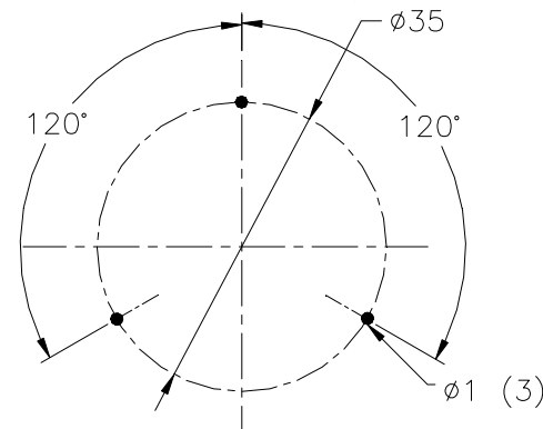
P.C. PIN HOLE PATTERN
