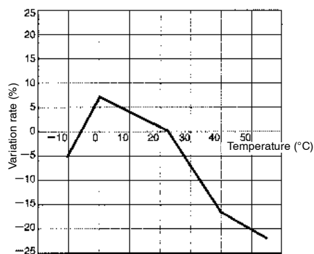
E2J-W10MA
