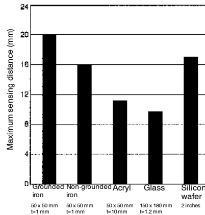
E2J-W20MA
