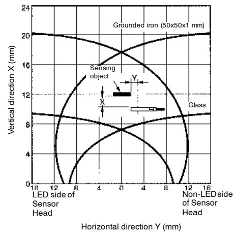
E2J-W20MA
