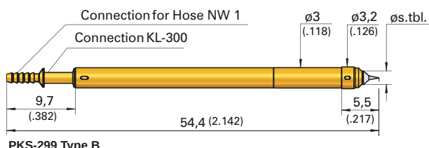
PKS-299 Type B
