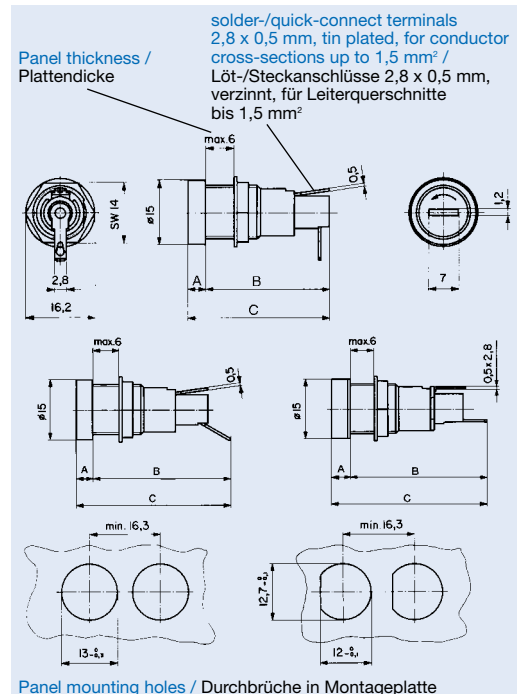
Panel mounting holes / Durchbrüche in Montageplatte
