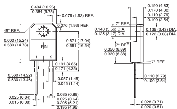
ITO-220AC
