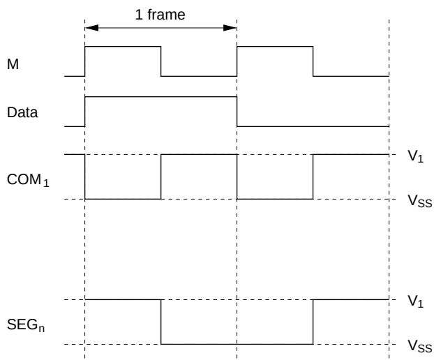
Figure 12-11 (d) Waveforms at Static Duty
