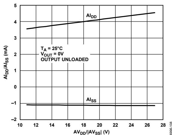
Figure 8. A_{II}/A_{ISS} vs. AV_{DD}/AV_{SS}
