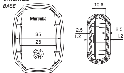
UNTERTEIL BASE
