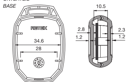
UNTERTEIL BASE
