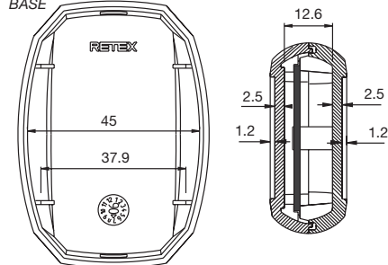
UNTERTEIL BASE
