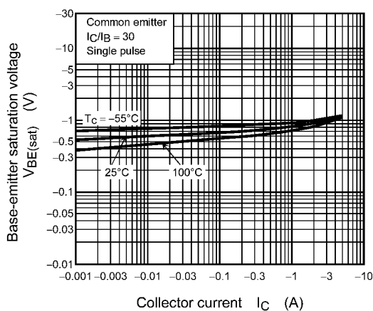
Fig. 7.4 V_{BE(sat)} - I_C
