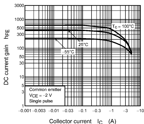
Fig. 7.2 h_{FE} - I_C
