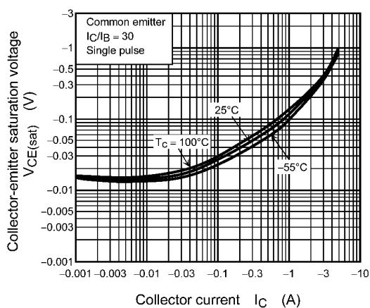
Fig. 7.3 V_{CE(sat)} - I_C
