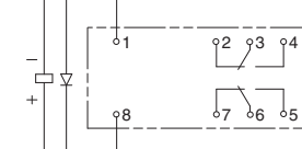
G2R-2-SN, G2R-2-SNI (DC)
