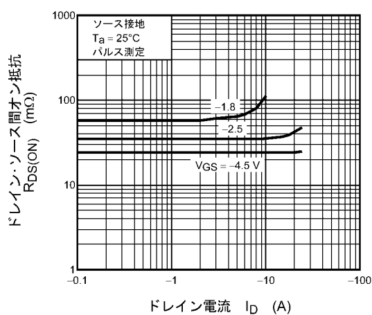
図 8.5 R_{DS(ON)} - I_D
