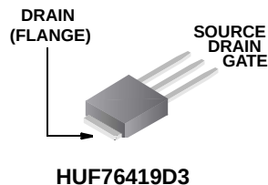
JEDEC TO-251AA
