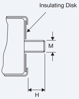
ALS35 Stud Mounting
