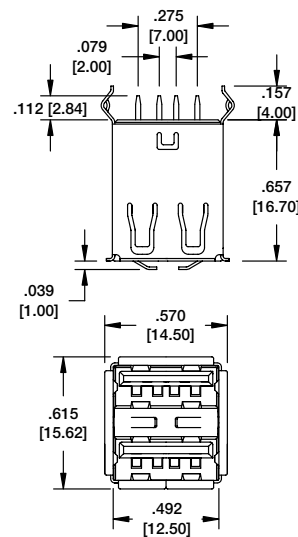
USB-A-Q-RA
