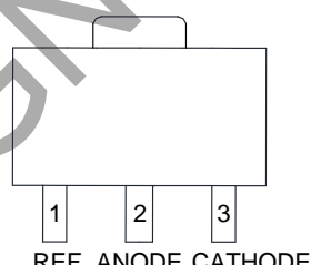
SOT-89 (Option 2)
