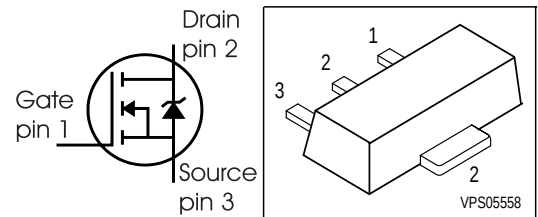
P-SOT89-4-2
