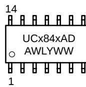
SOIC-14 D SUFFIX CASE 751A
