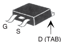
TO-263 (IXTA)
