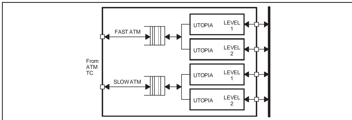
Figure 8 : Interface Module
