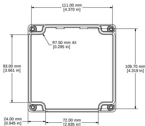
LID - INSIDE
