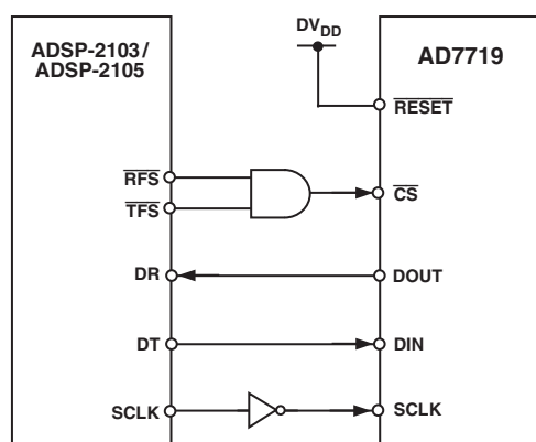
Figure 14. AD7719-to-ADSP-2103/ADSP-2105 Interface
