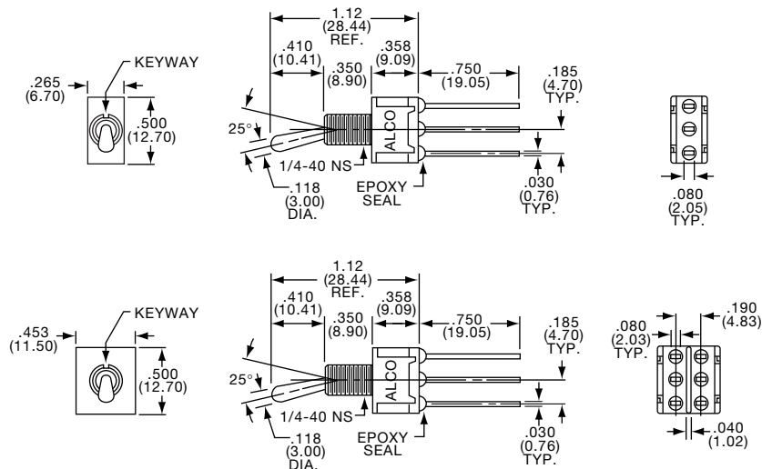
SPDT/DPDT
